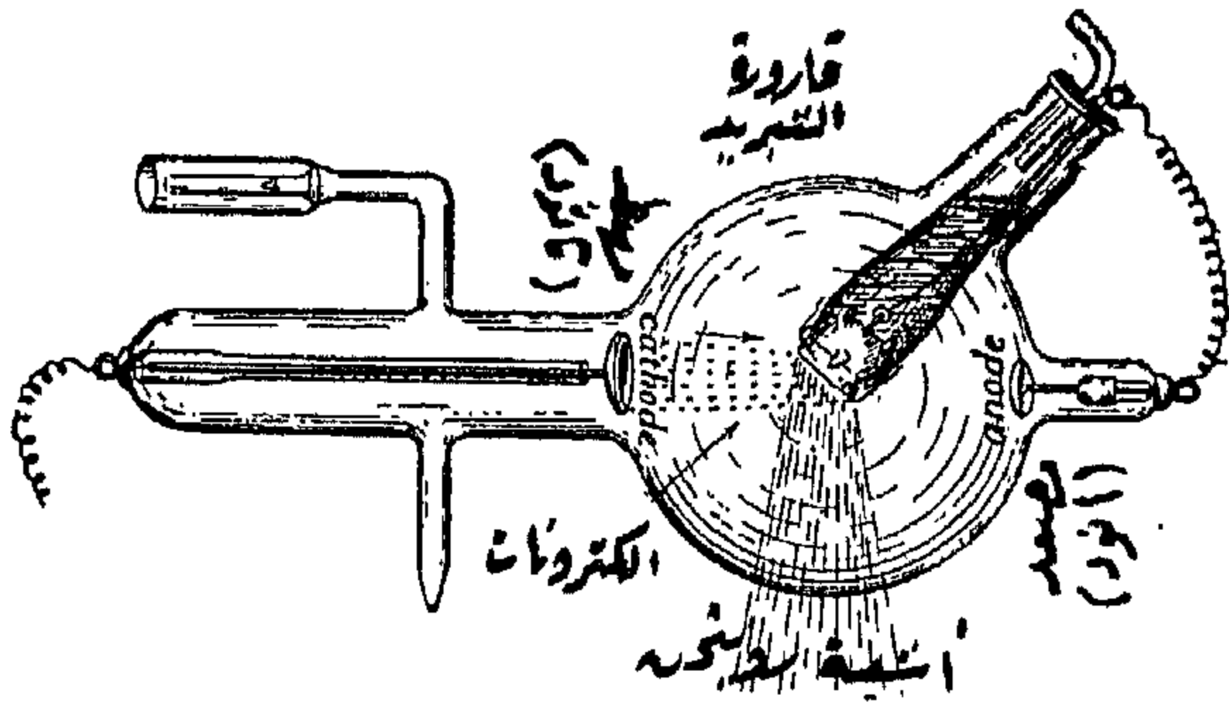
(شكل ١٠٣) أنبوبة أشعة روننتجن
